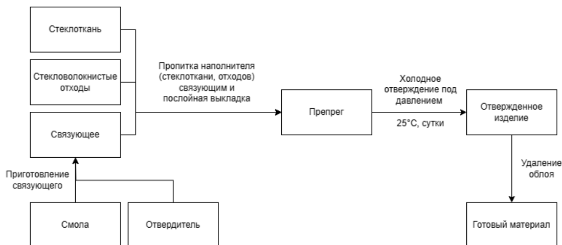
Рис. 9. Блок-схема технологии получения пресс-материалов с эпоксидной смолой
