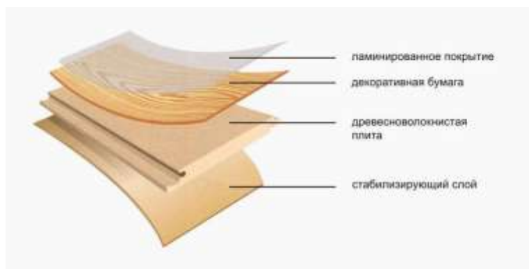
Рис. 1. Строение ламинированного напольного покрытия
