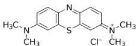
Рис. 2. Структурная формула метиленового голубого
