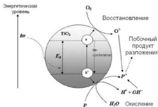
Рис. 1. Принцип фотокаталитического действия наноразмерного TiO 2
