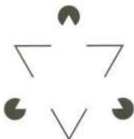
Рис. 1. Треугольник Канижа
