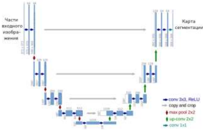
Рис 5. Архитектура U-Net
